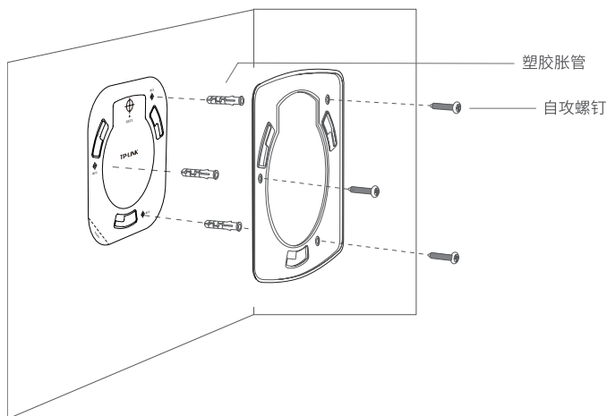
图3-10 固定安装架到墙面示意图
